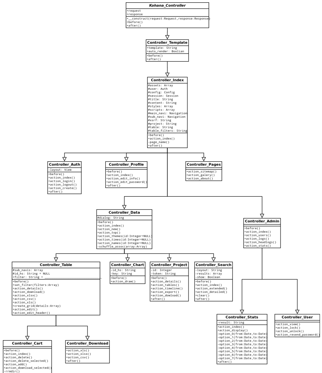
Abb.5 Controller Klassendiagramm
