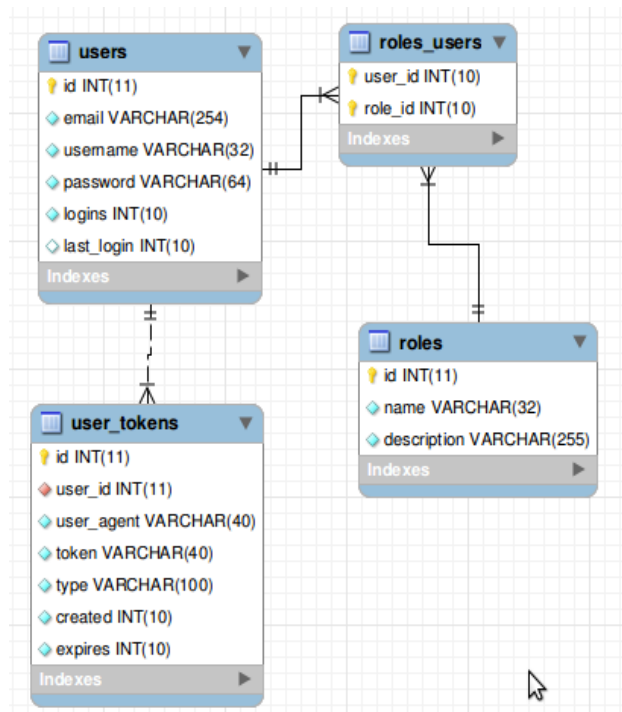
Abb.4 ERD RBAC
